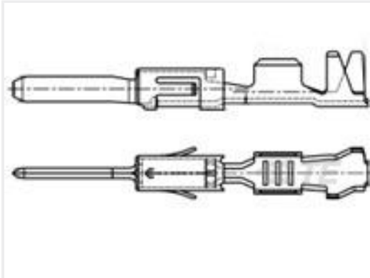
TE Part #963904-3 TAB A 1.6x0.6 CONTACT CS SWS Au
