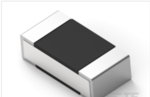
TE Part #3-2176306-3 RP 1E 0.1W 2K49 0.1% 25PPM 5K RL
