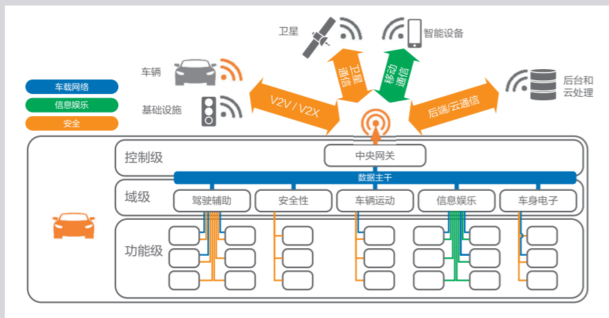
图 2: 互联车辆可能的系统架构
