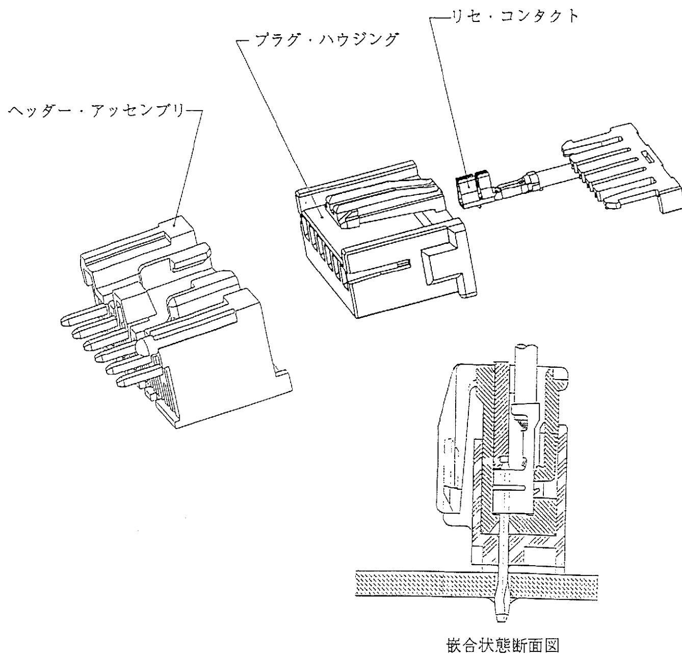
Fig. 2 電線対基板接続タイプ
