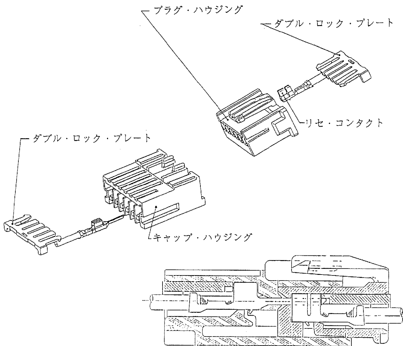
嵌合状態断面図
