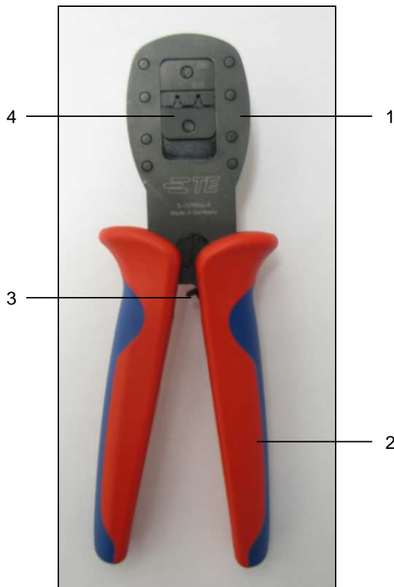
Abb. 1: Handzangenkomponenten
