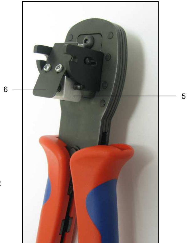
Abb. 2: Handzangenkomponenten
