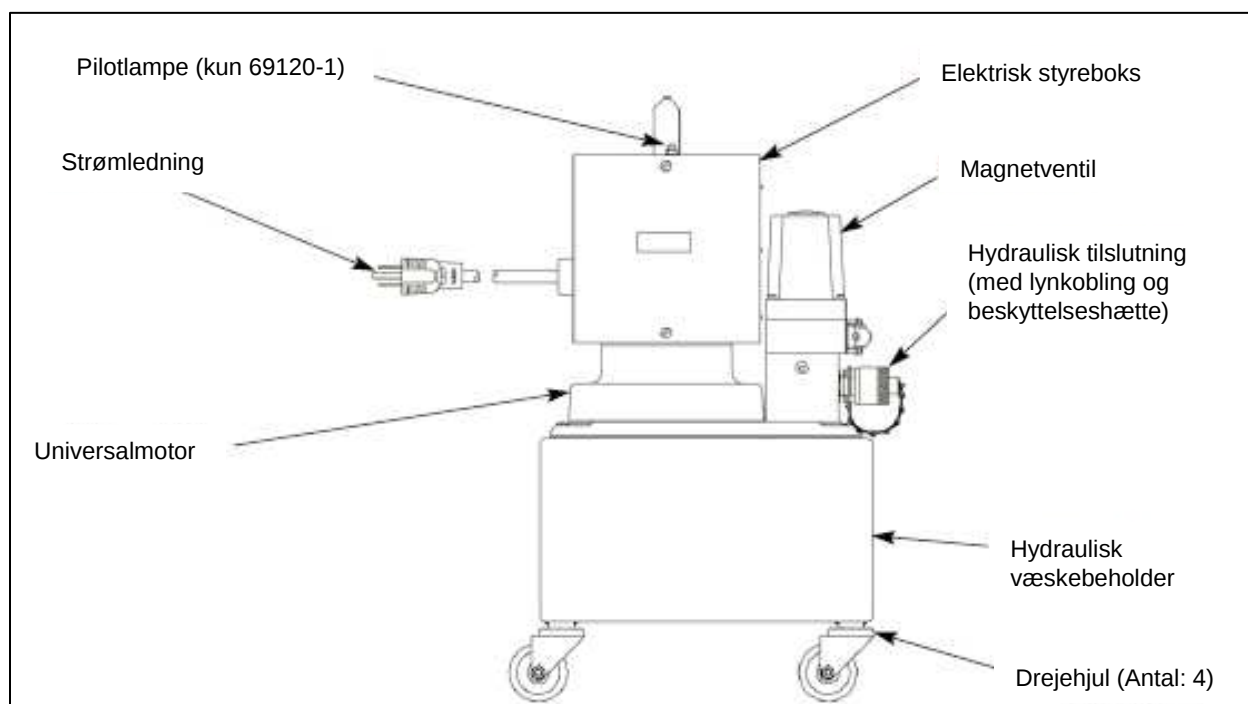
Figur 1: Elektrisk hydraulikpumpe til tung belastning
