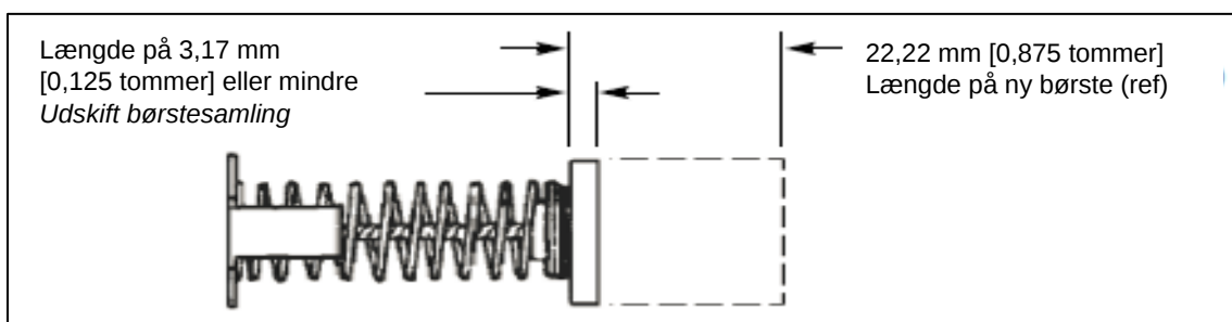
Figur 10: Kontrol af børstesamling på universalmotor
