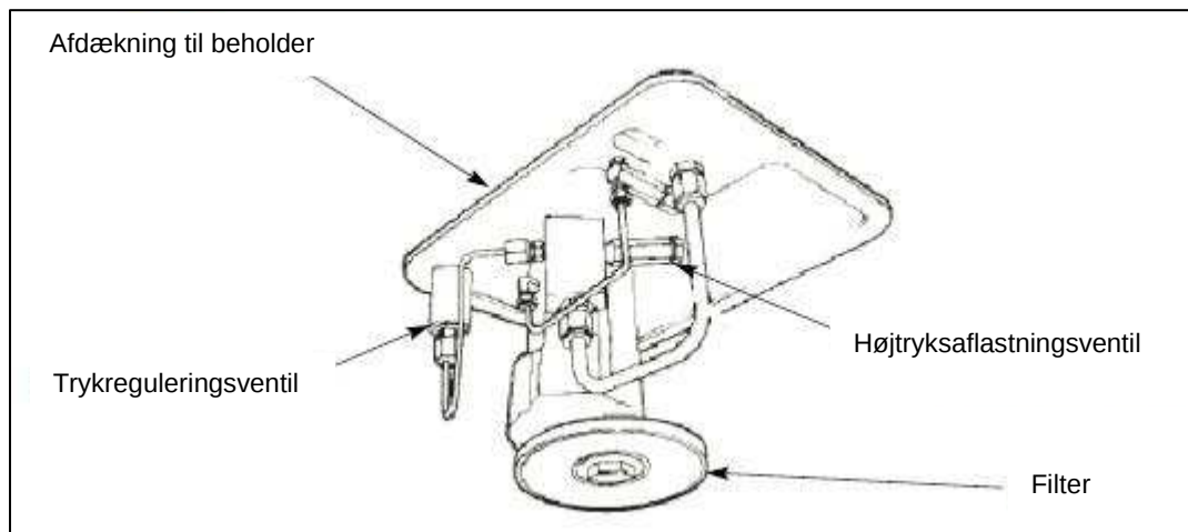
Figur 8: Motor- og pumpesamling
