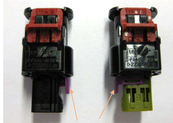
Bild 1: 2pol., HPF 1.2, Flachkontaktgehäuse, radialdicht
