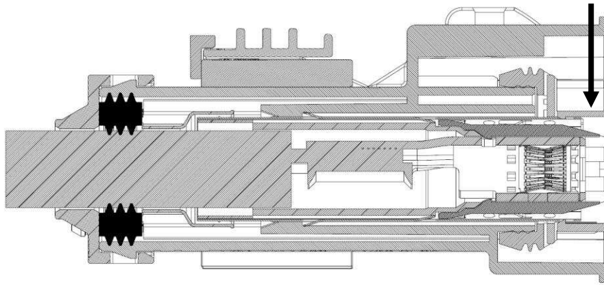
Figure 20: Cross section through locking latch Querschnittsdarstellung durch die 2.Kontaktsicherung
