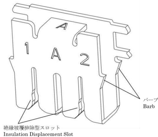
A. Terminal
