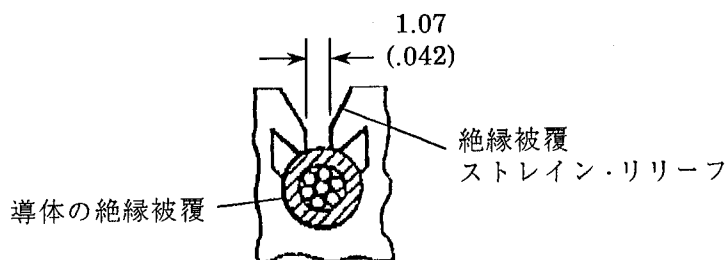
Fig. 8 ストレイン・リリーフ
