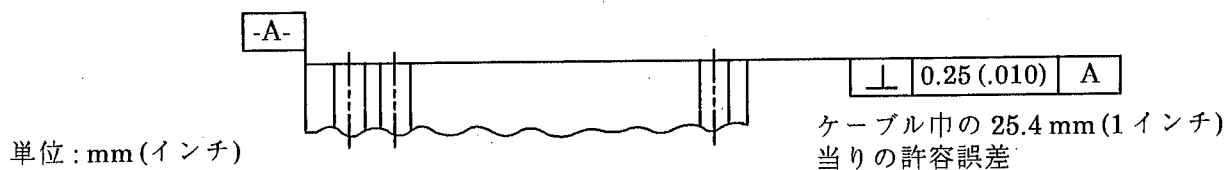
Fig. 3 ケーブル端縁部の切断直角度
