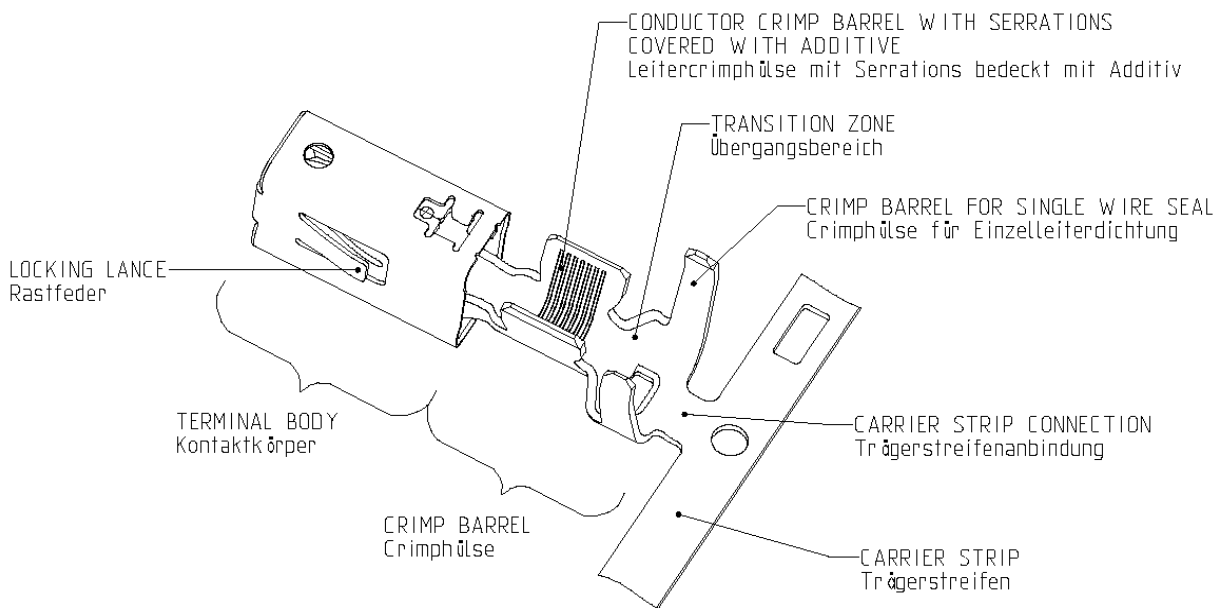
Figure 2: Terminals with crimp for single-wire-seals and aluminium wires / Bild 2: Kontakte mit Crimp für Einzelleiterdichtungen und für Aluminiumleitungen
