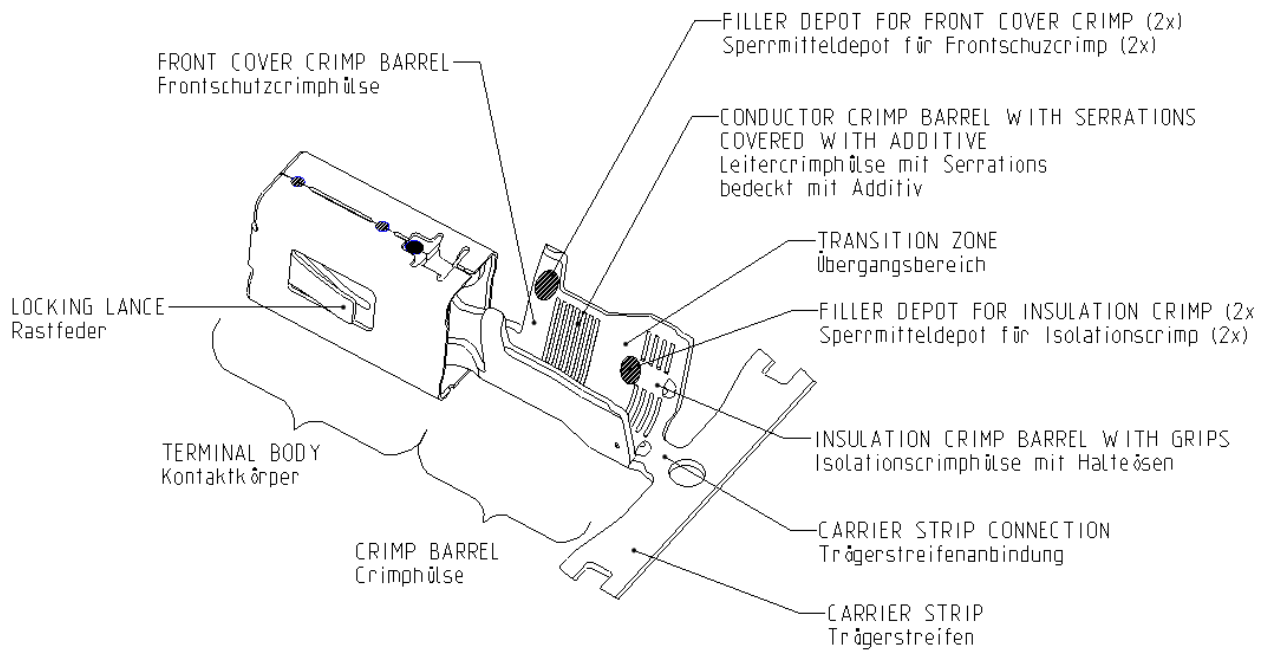
Figure 1: Terminals with TE self-covering F-crimp barrels for aluminium wires / Bild 1: Kontakte mit TE selbstschützenden F-Crimphülsen für Aluminiumleitungen
