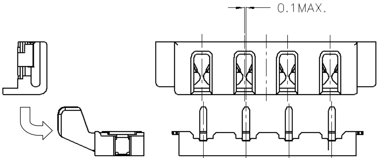
Fig.4-1 ピッチ方向の位置ずれ許容量(耐久性試験) Fig.4-1 Displacement allowance for durability test
