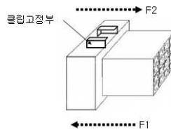
<그림 5-9: 하우징 클립간 삽입/이탈력>
