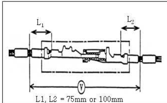
&lt; 그림 5-4 : HARNESS 對 HARNESS &gt;
