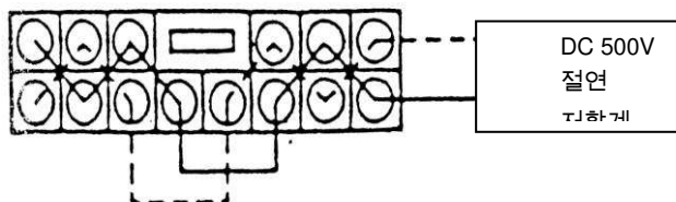
&lt;그림 5-6 : 인접단자 상호간&gt;
