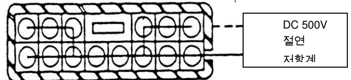
&lt;그림 5-7 : 인접단자와 HSG 표면간&gt;
