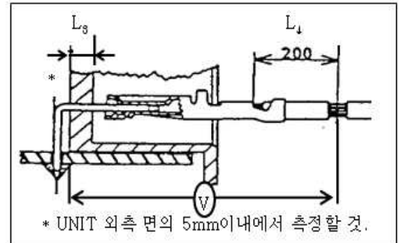
&lt; 그림 5-5 : HARNESS 對 UNIT &gt;
