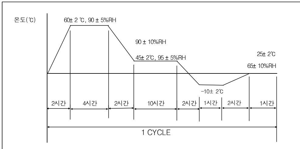
<그림 6-3 : 시험 PATTERN >
