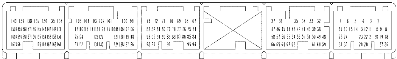
Fig.13 167 極回路番号
