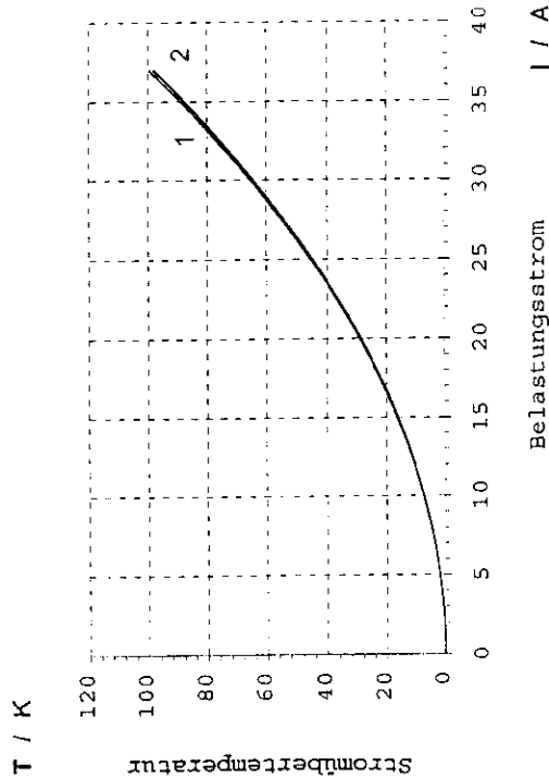
Stromerwärmung
