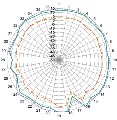
XZ-Plane Gain
