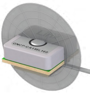
XZ-Plane Gain
