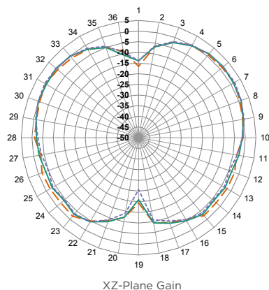
XZ-Plane Gain
