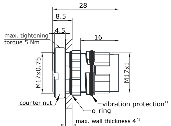
Main Dimensions receptacle
