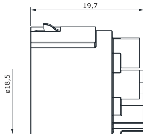
Hauptabmessungen Isolierkörper
