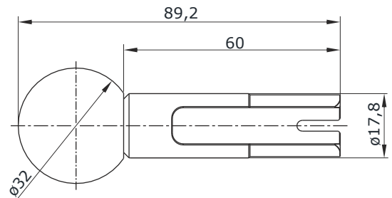
Hauptabmessungen Montagewerkzeug
