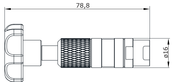
Hauptabmessungen Ausbauwerkzeug
