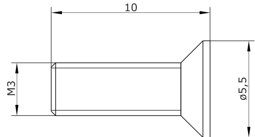
Hauptabmessungen Schraube
