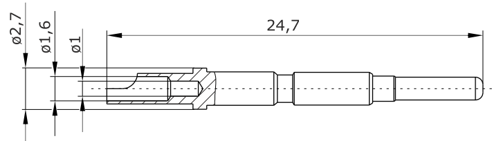
Hauptabmessungen Kontaktstift
