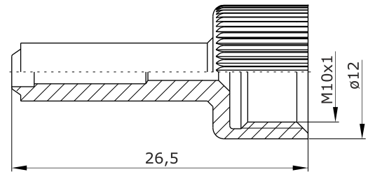
Hauptabmessungen Ausbauhülse
