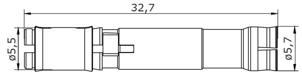
Hauptabmessungen Ethernet
