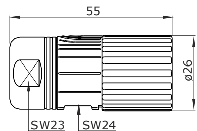
Hauptabmessungen Stecker
