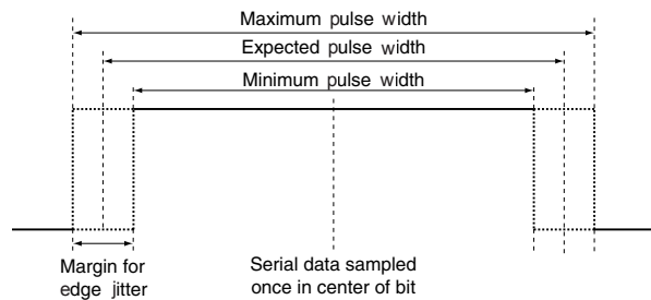
Figure 3: Edge Jitter
