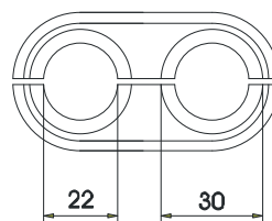
Kabelzugang
