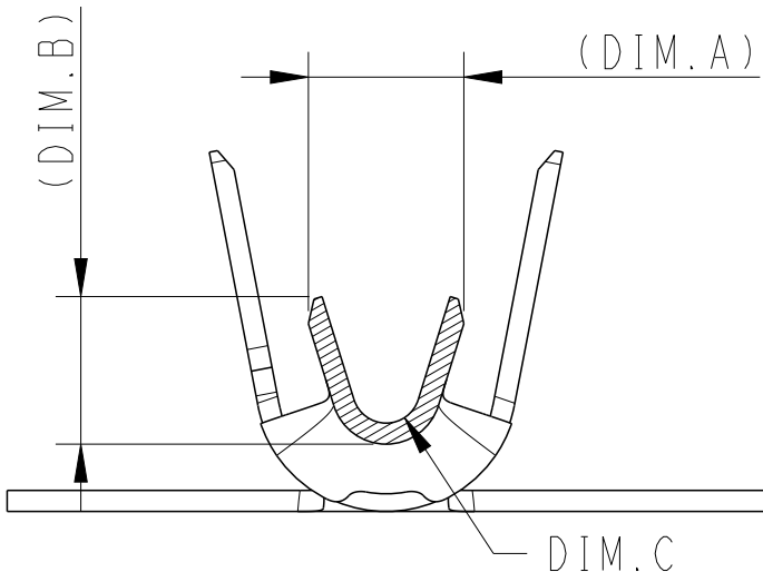
SECTION D-D SCALE 10:1
