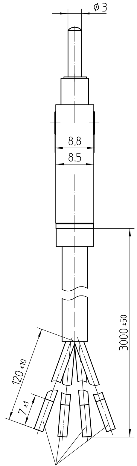
Aderendhülle DIN 46 228
