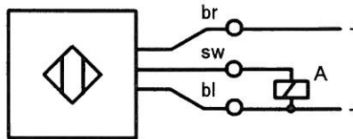
Schaltbild:
