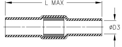
3) SOLDER SLEEVE, Qty/kit.: 2
