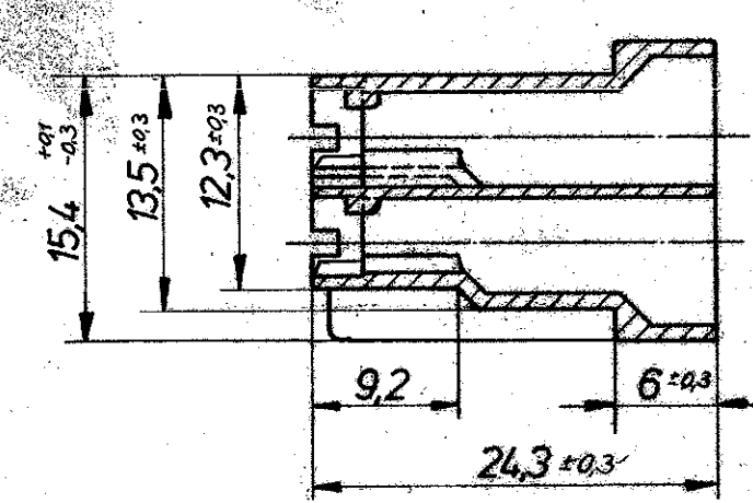
Schnitt A-A
