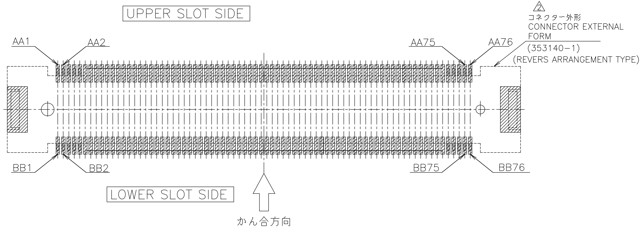
F.P.C. コネクター基板パターン F.P.C. CONNECTOR P.C.BOARD LAYOUT
