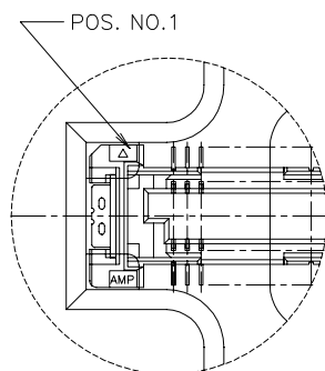
DETAIL E (SCALE 4:1)
