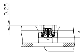
D-D (SCALE 2:1)
