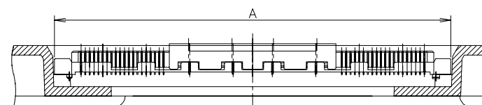
C-C (SCALE 2:1)
