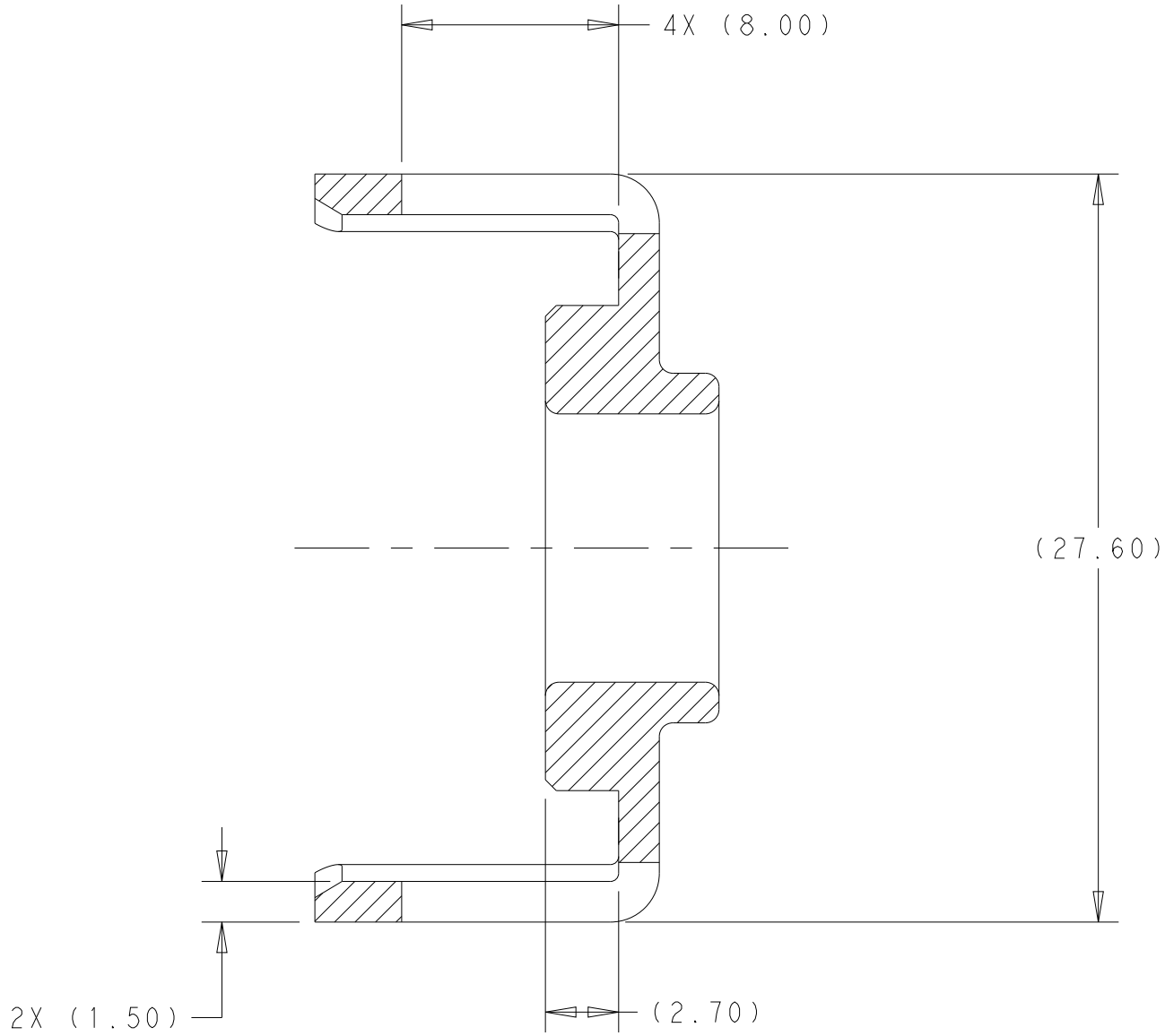
SECTION D-D
