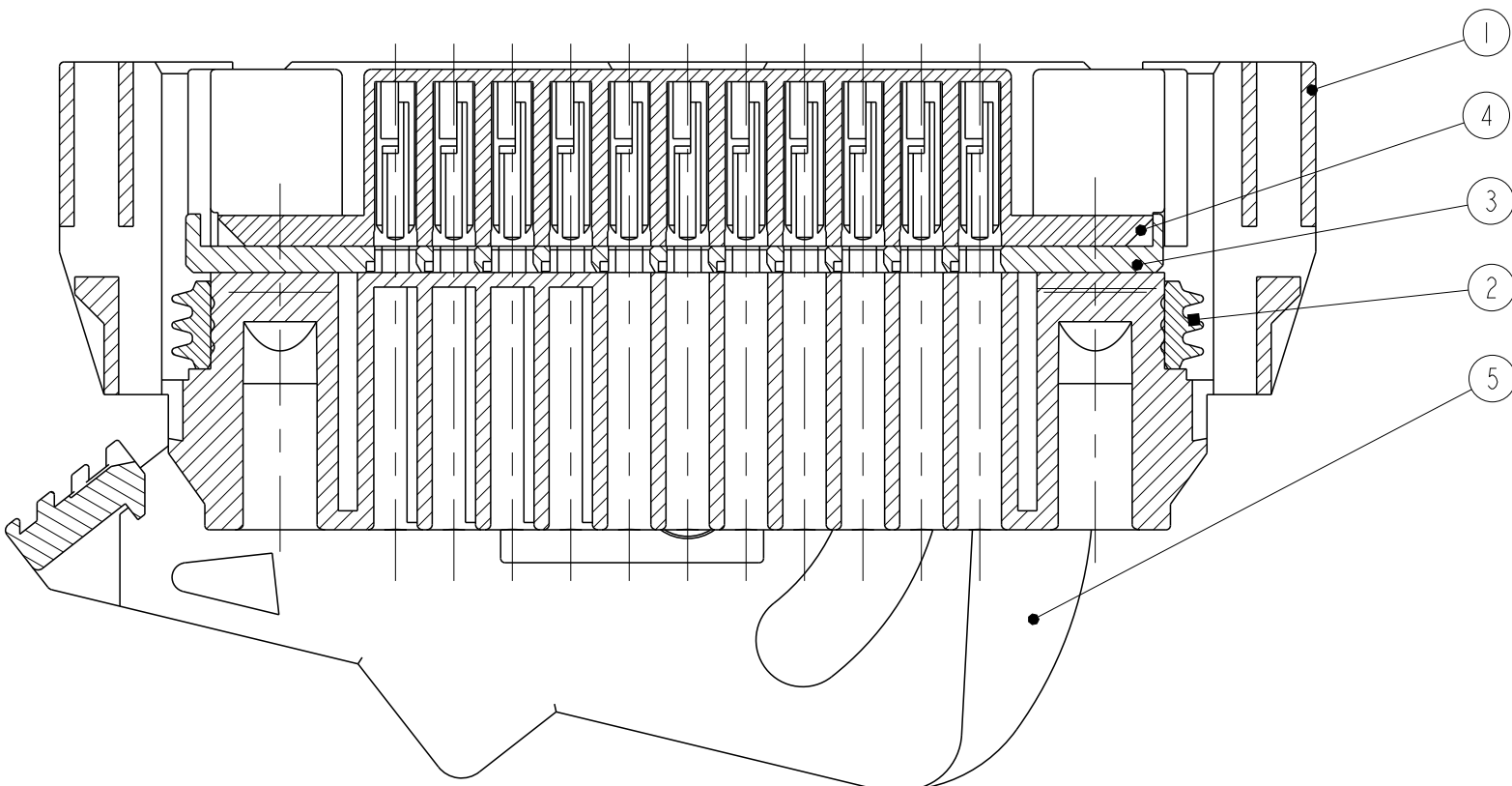
SECTION A-A
