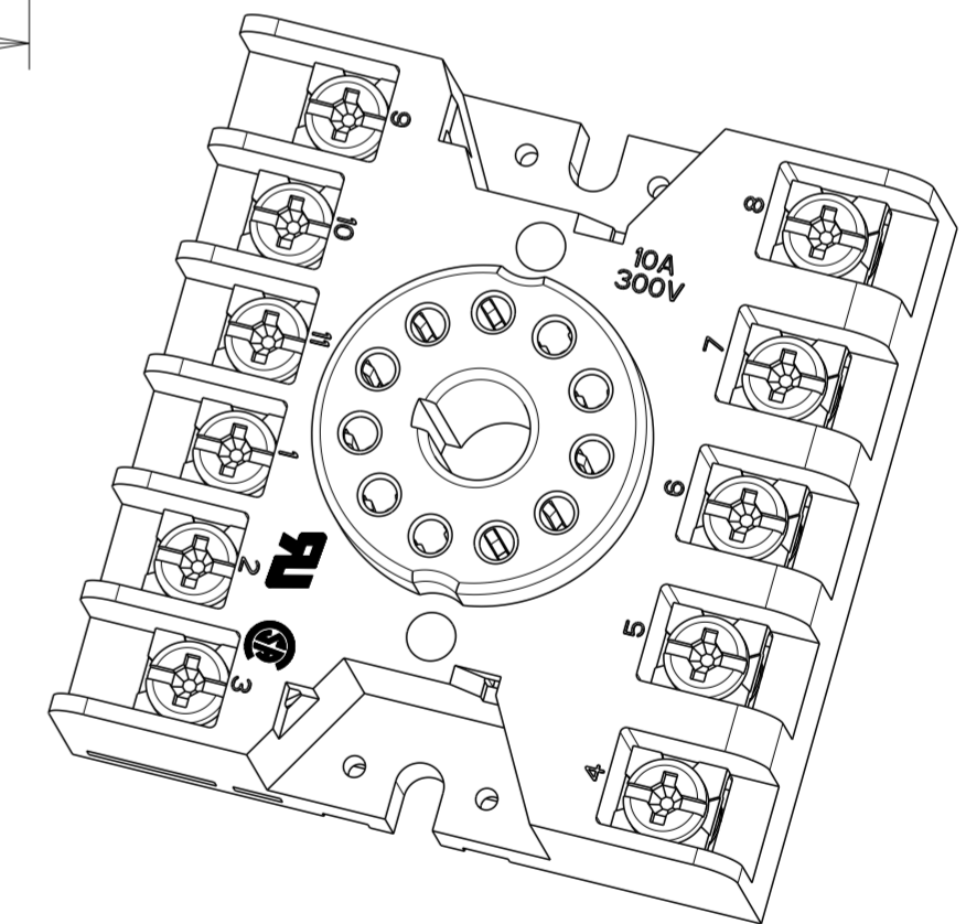
SCALE 3:2
