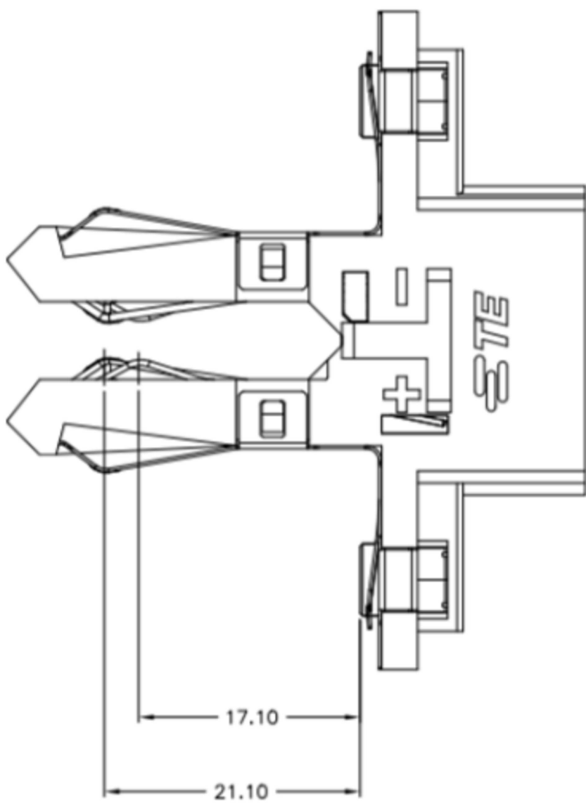
FIN SIDE
