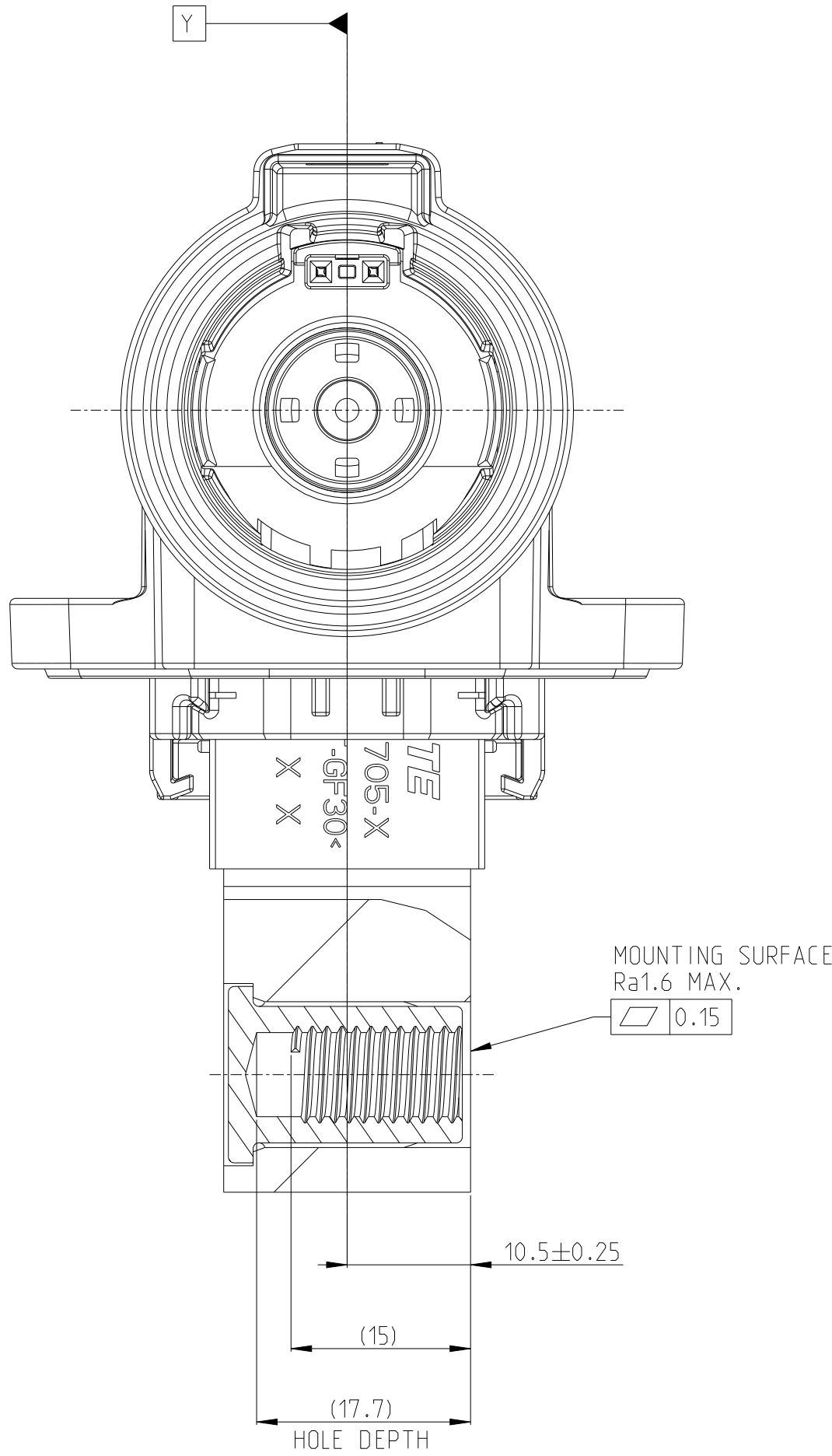
SECTION D-D
