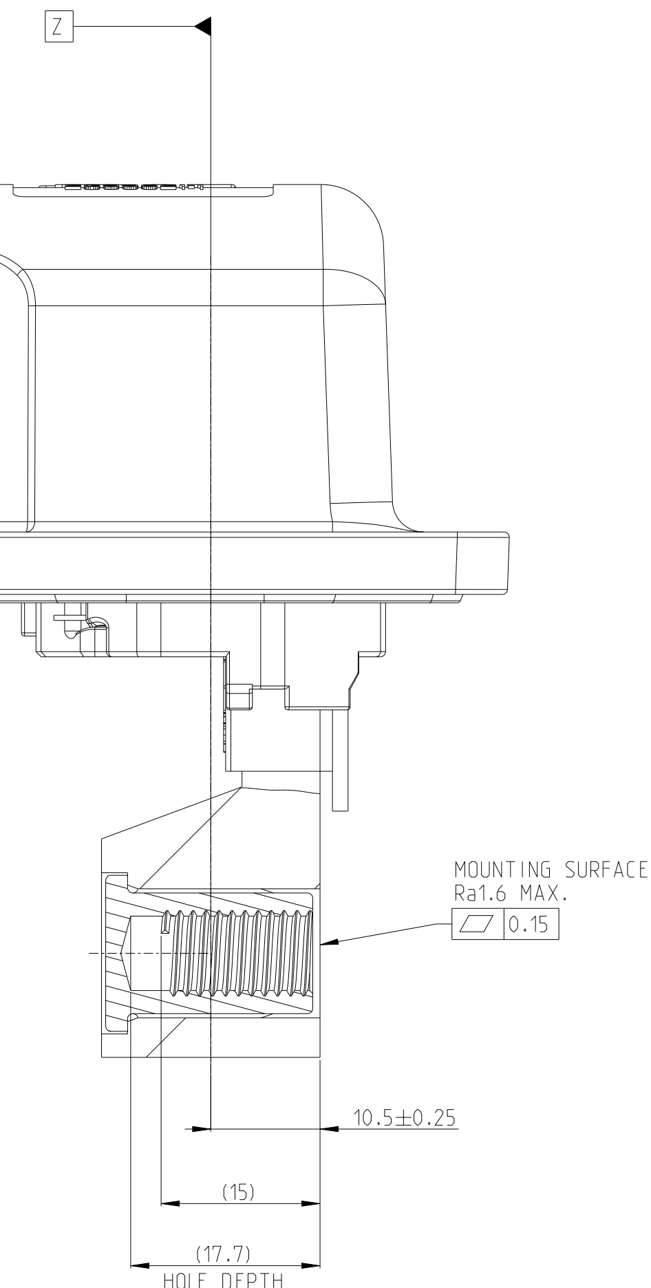
SECTION A-A
