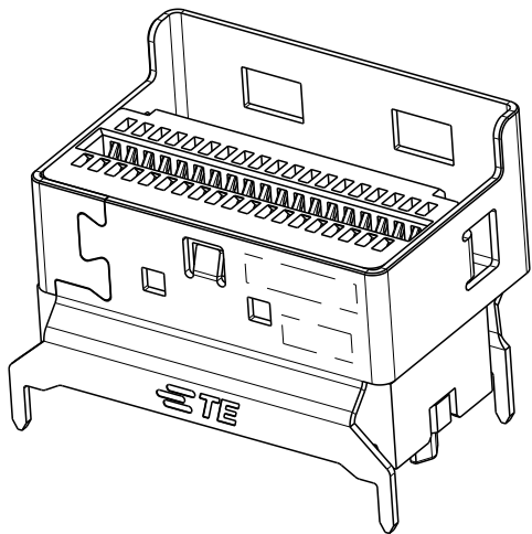
W/O DUST CAP SCALE 4:1
