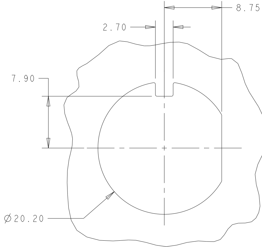
RECEPTACLE CUTOUT SCALE 3:1
