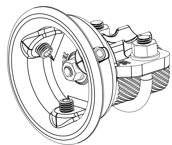
Cable ø15/16 to 1 11/16
