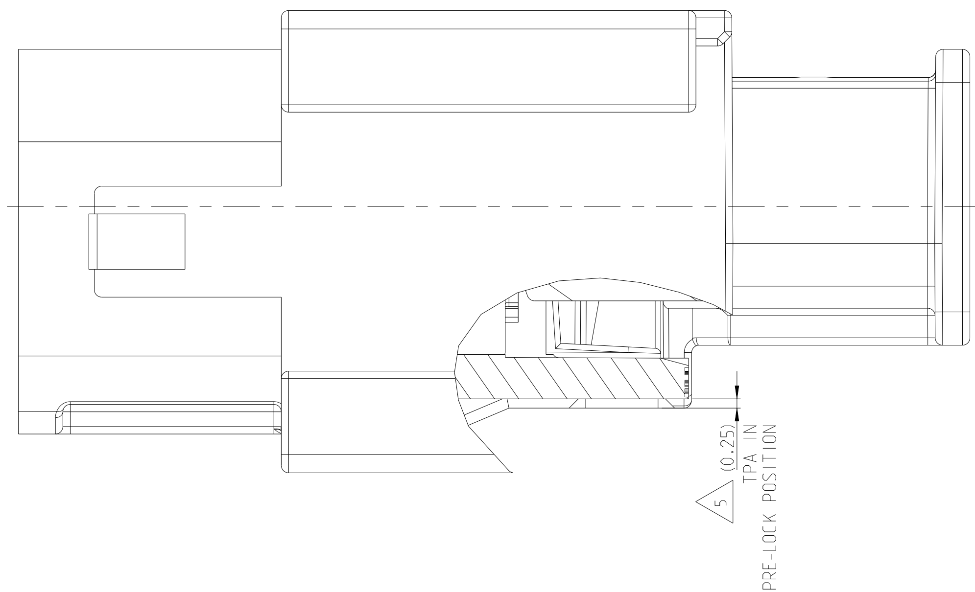
SECTION A-A
