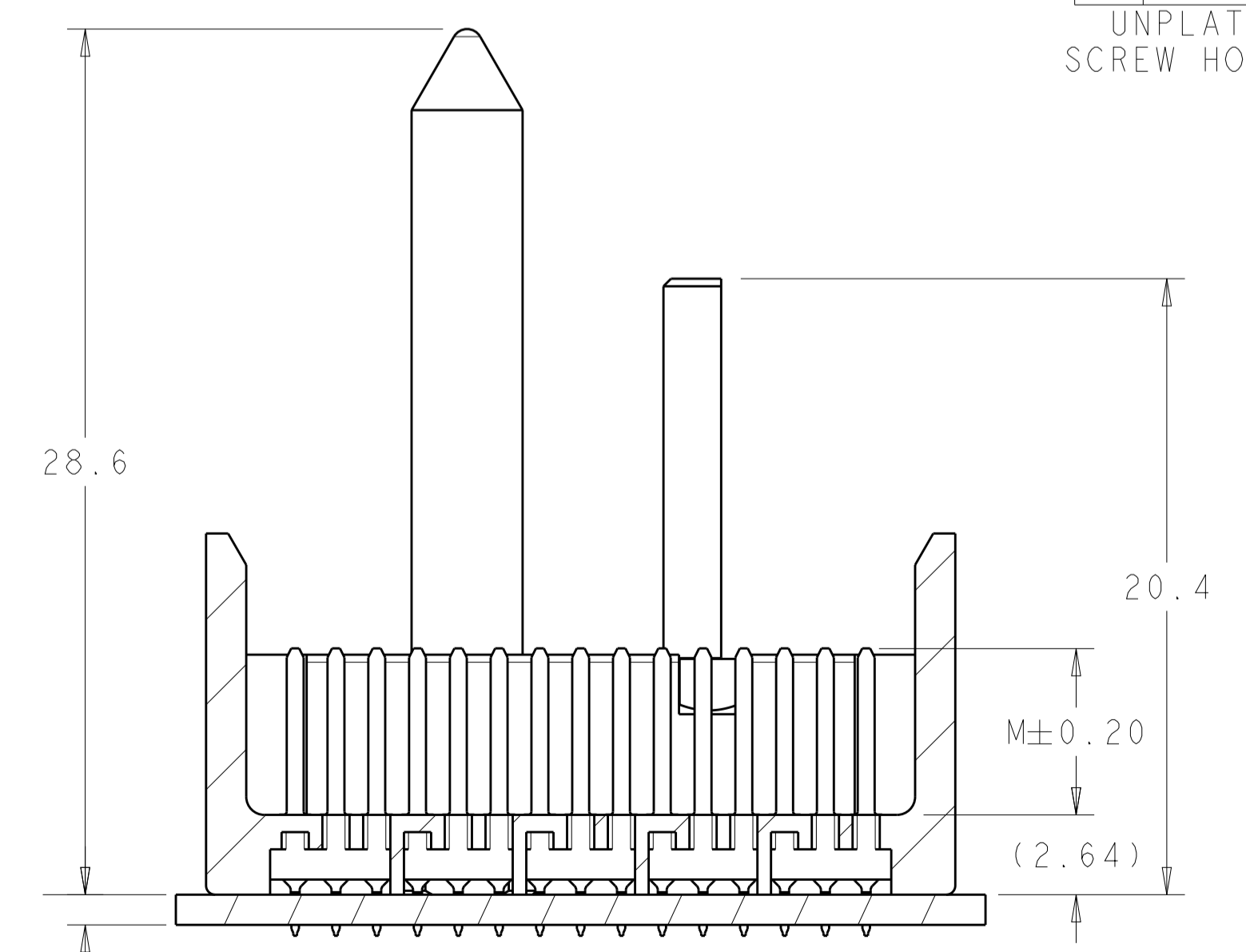
SECTION A-A
