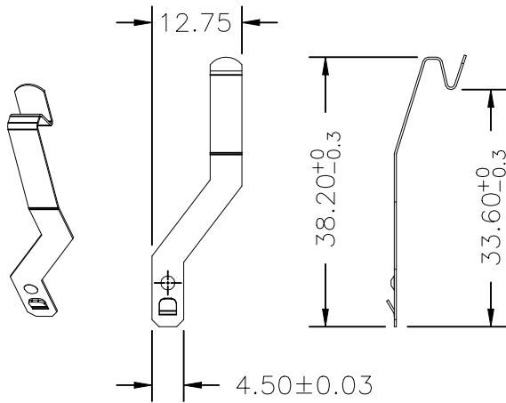
DIN type clip 2071566-7 PT28D00
