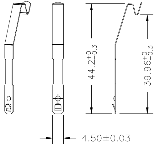
DIN type clip 2071566-9 PT28D01
