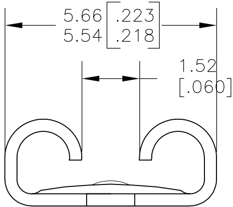
VIEW A-A
