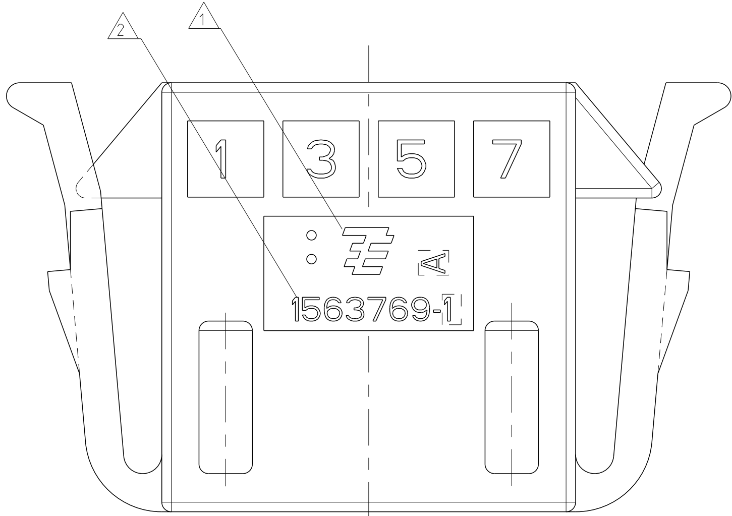
VIEW X ANSICHT
