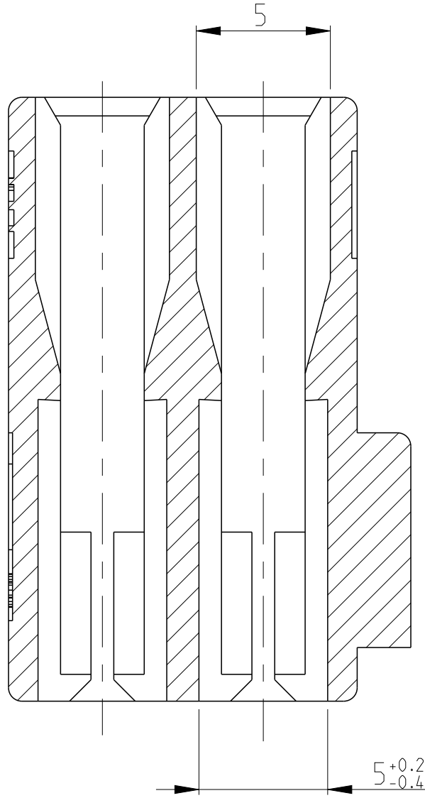
SECTION A-A Schnitt
