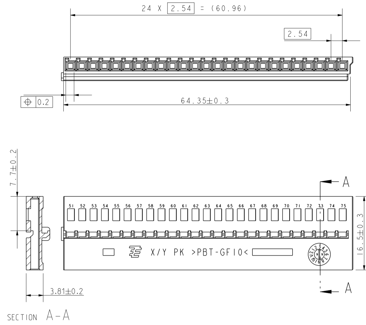
SECTION A-A
